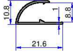
5320 0.115 kg/m
