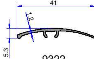
9322 0.156 kg/m
