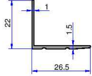
4995 0.153 kg/m
