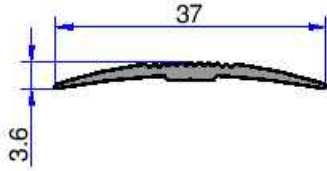
6505 0.147 kg/m
