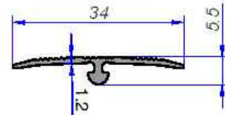
10-2723 0.127 kg/m
