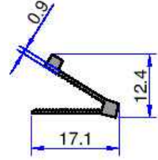
3852 0.089 kg/m
