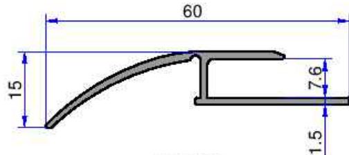
5888 0.347 kg/m
