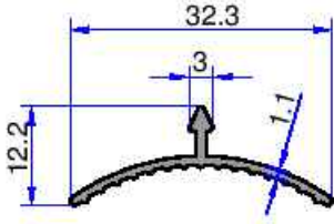
5305 0.137 kg/m
