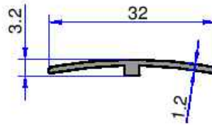
5267 0.120 kg/m
