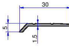
4997 0.116 kg/m
