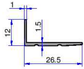
4996 0.126 kg/m
