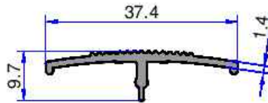
5088 0.207 kg/m
