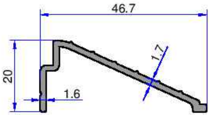
11163 0.321 kg/m
