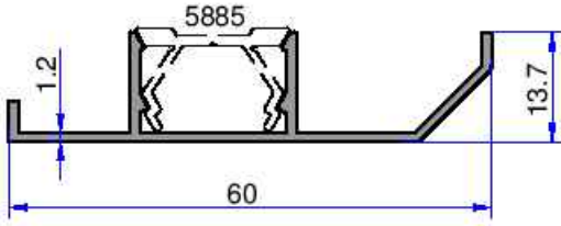
5022 0.328 kg/m
