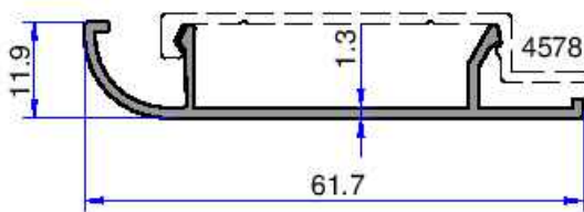
4577 0.323 kg/m
