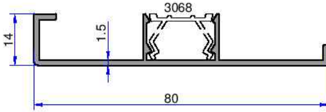
10265 0.496 kg/m
