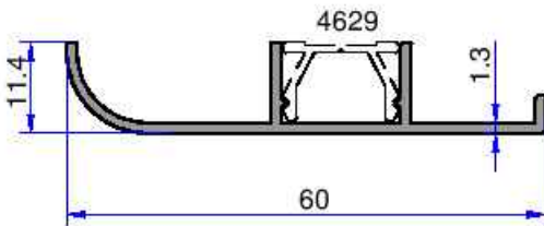
4628 0.317 kg/m
