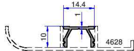
4629 0.101 kg/m
