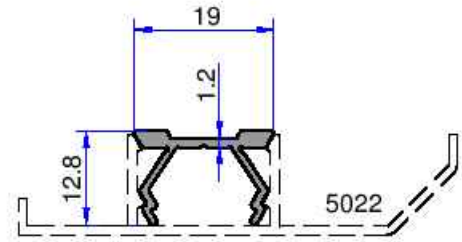
5885 0.153 kg/m
