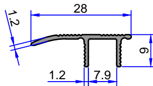
10-2713 0.127 kg/m
