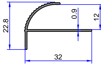
6126 0.160 kg/m
