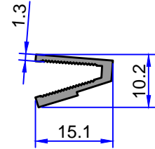
3867 0.120 kg/m
