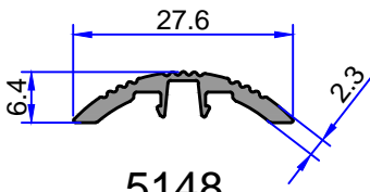
5148 0.157 kg/m
