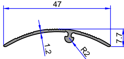
10-2721 0.176 kg/m
