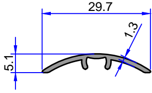
9427 0.121 kg/m
