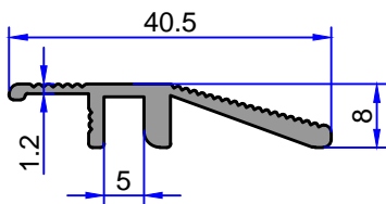
5282 0.286 kg/m
