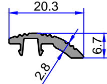
5149 0.134 kg/m
