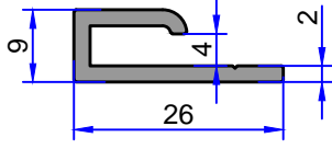
5559 0.244 kg/m
