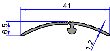
10-2722 0.157 kg/m
