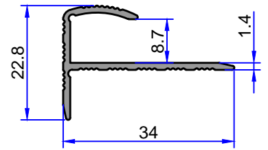
10-2708 0.230 kg/m
