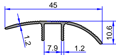
10-2712 0.186 kg/m
