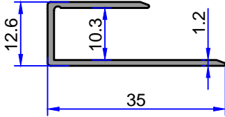
9007 0.204 kg/m
