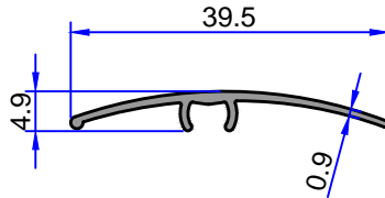
10108 0.138 kg/m
