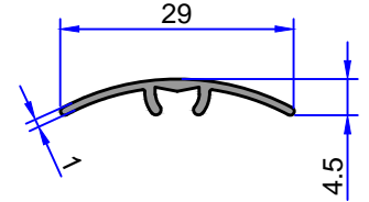
5381 0.107 kg/m
