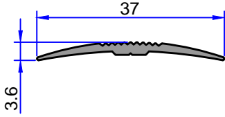
6505 0.147 kg/m
