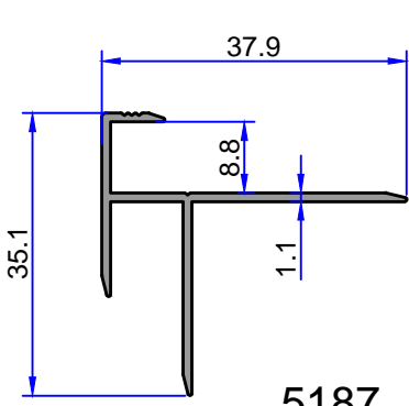
5187 0.259 kg/m
