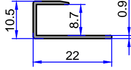
5285 0.097 kg/m
