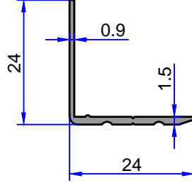
5188 0.143 kg/m
