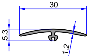
4999 0.116 kg/m
