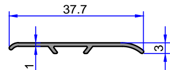
1706 0.117 kg/m
