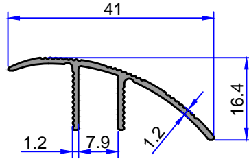
10-2714 0.202 kg/m
