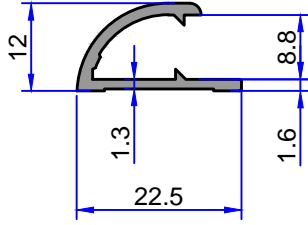
3883 0.181 kg/m
