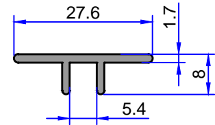
3235 0.173 kg/m
