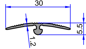
10-2716 0.114 kg/m
