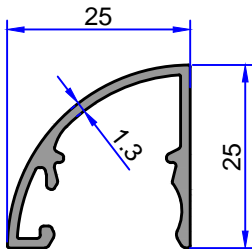
10448 0.291 kg/m
