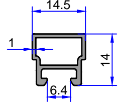
11051 0.163 kg/m
