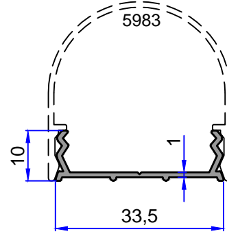
5982 0.155 kg/m
