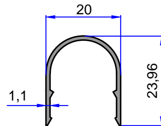
3067 0.173 kg/m
