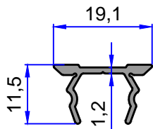
5889 0.132 kg/m
