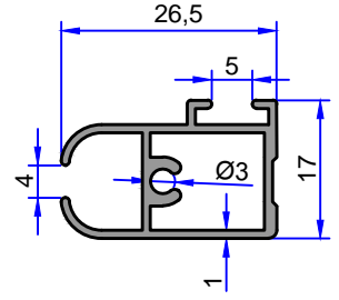
3565 0.287 kg/m
