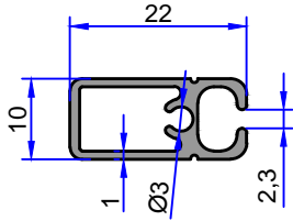
1501 0.213 kg/m
