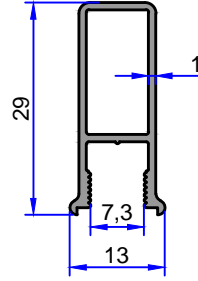
1529 0.220 kg/m
