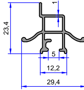
4283 0.255 kg/m
