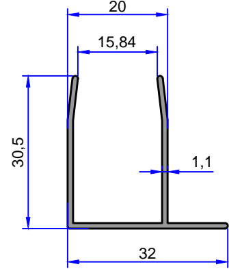
11150 0.270 kg/m
