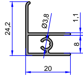
6611 0.227 kg/m
