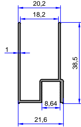
11574 0.297 kg/m
