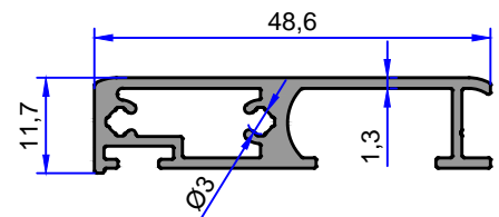
12148 0.480 kg/m
