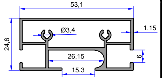
11988 0.710 kg/m
