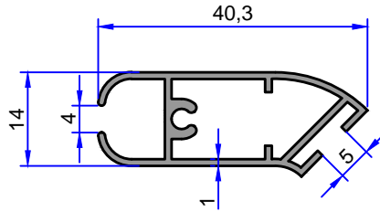
3567 0.336 kg/m
