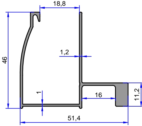
11268 0.630 kg/m
