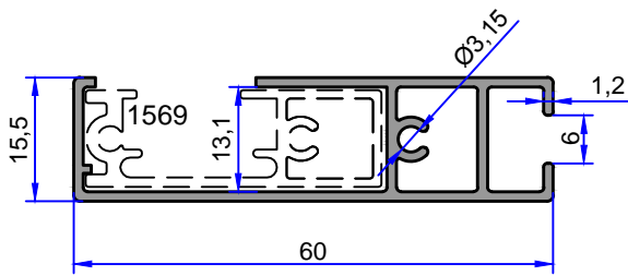
1568 0.508 kg/m
