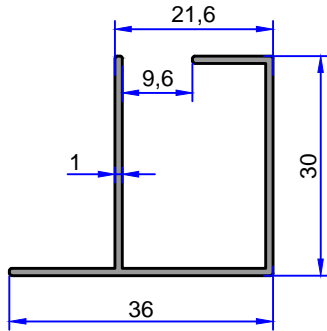
11966 0.281 kg/m
