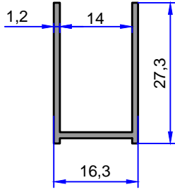
1551 0.214 kg/m
