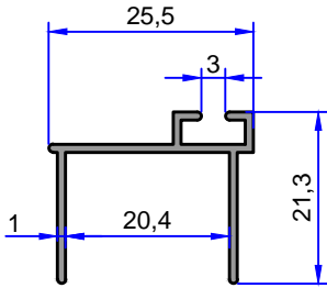
1494 0.191 kg/m
